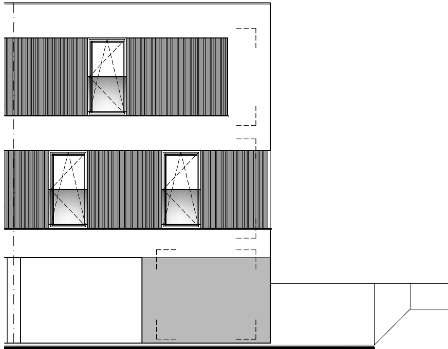
LOT 01 VOORGEVEL
