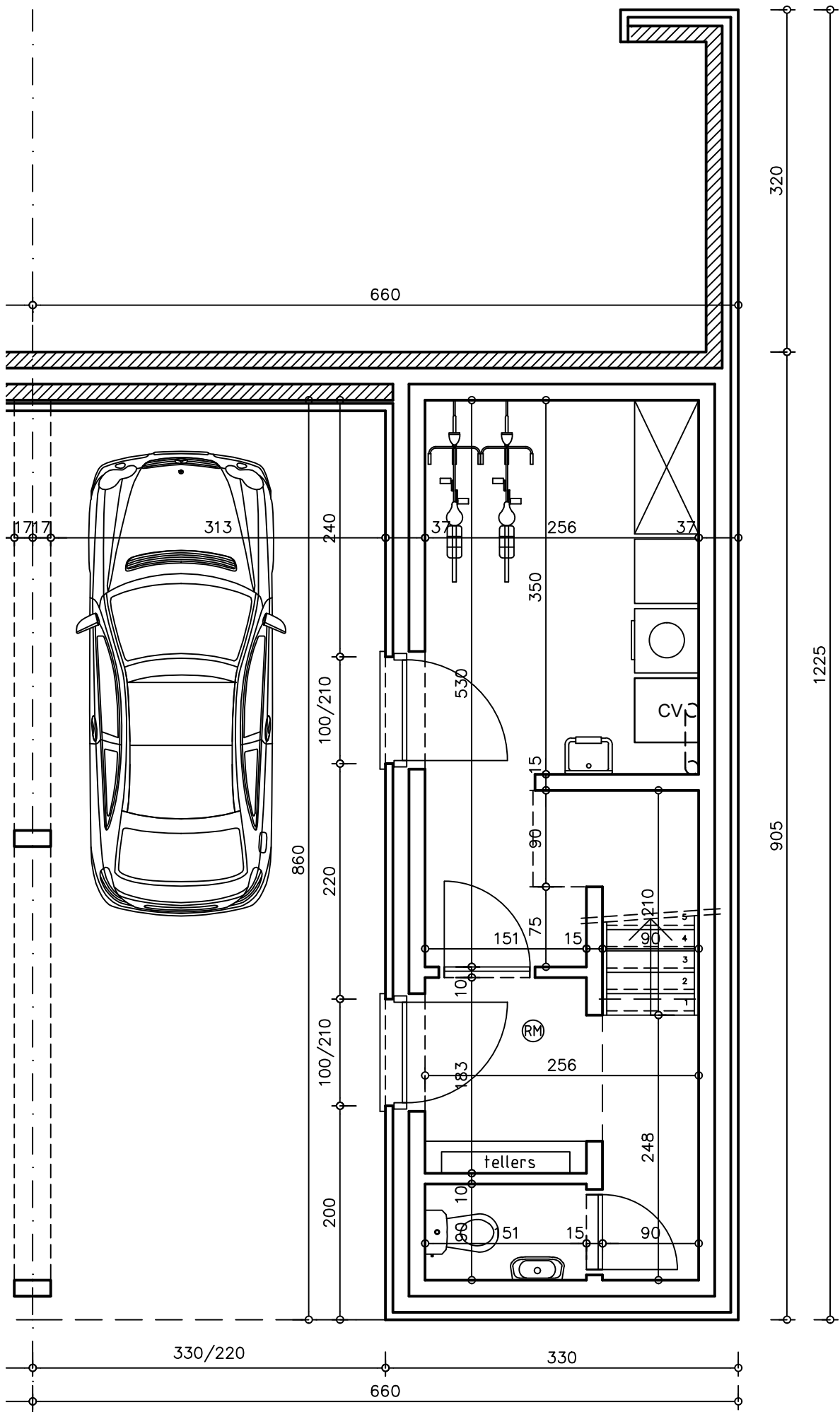
LOT 01 GELIJKVLOERS
